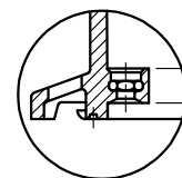
M4 ボス部 詳細図
